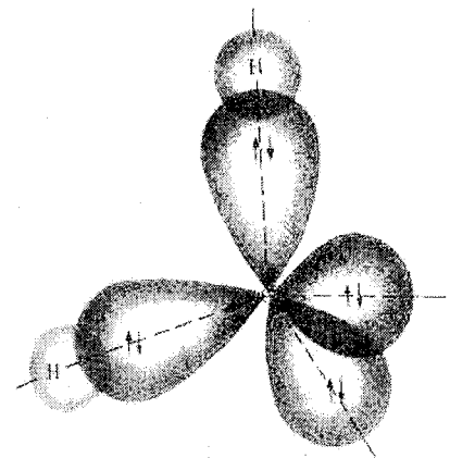
H 2 O
